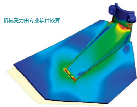
• 桨叶的机械力学分析
