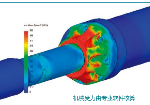
• 轴连接处机械力学分析
